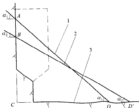
图 A.0.1 岩壁梁层与岩壁梁锚杆关系图
