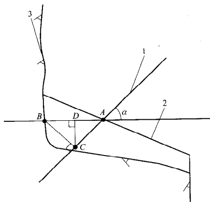
图 C.0.3 岩台超挖后 C 锚杆实际开孔孔位与设计孔位关系图
