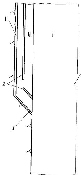
图 B.0.2 岩壁梁岩台垂直和斜孔 光面爆破示意图 (单位: cm)
